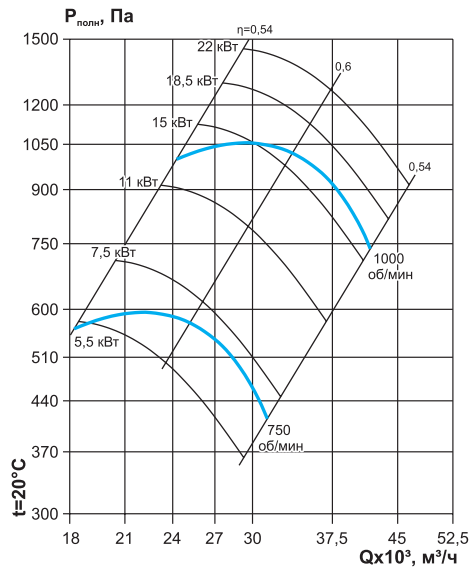
ВКР №10,0 (D=d0,95)
