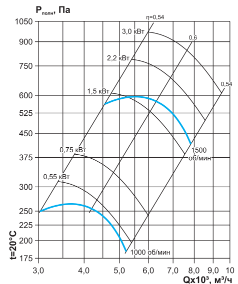
ВКР №5,0 (D=d0,95)
