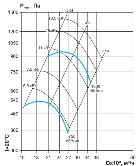
ВКР №10,0 (D=d0,9)
