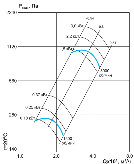
ВКР №3,15 (D=d1,0)
