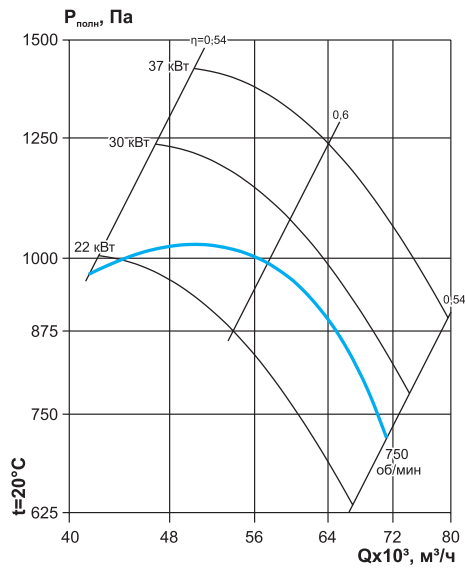
ВКР №12,5 (D=d1,0)
