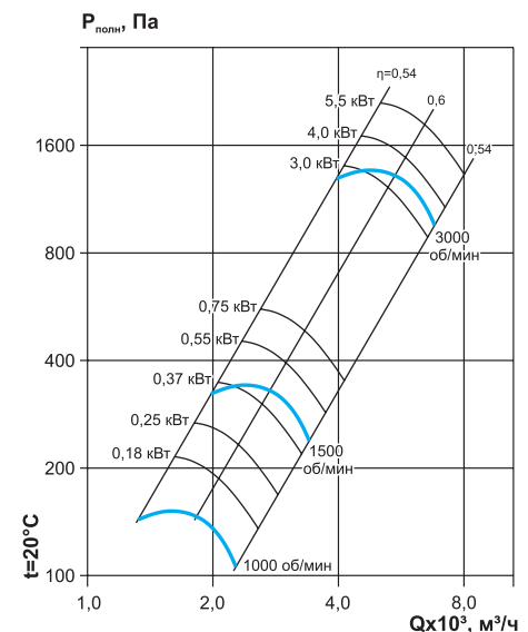
ВКР №4,0 (D=d0,9)
