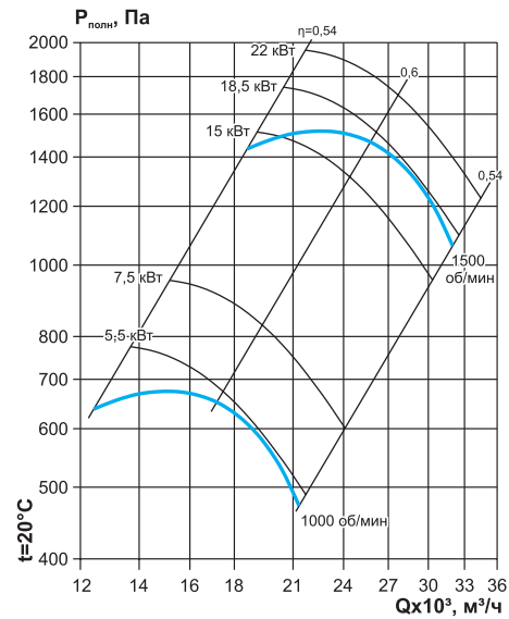
ВКР №8,0 (D=d0,95)
