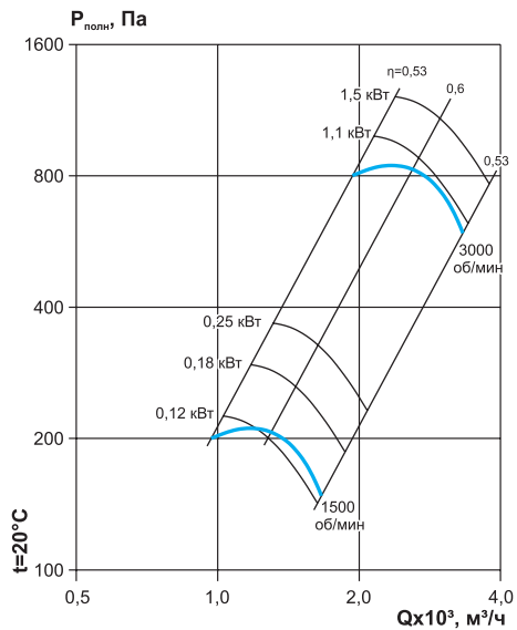
ВКР №3,15 (D=d0,9)
