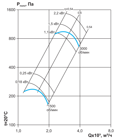
ВКР №3,15 (D=d0,95)
