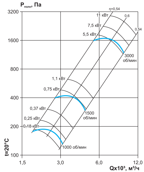
ВКР №4,0 (D=d1,0)
