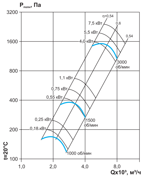
ВКР №4,0 (D=d0,95)
