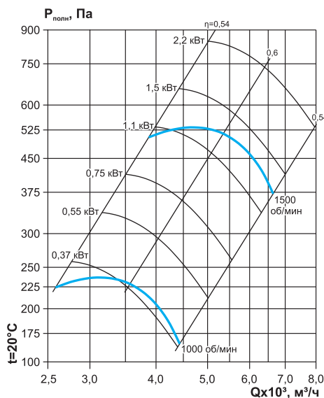
ВКР №5,0 (D=d0,9)
